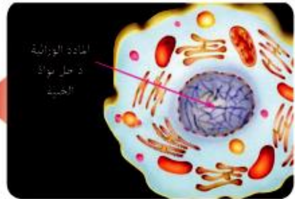
▲ شكل (١) الخلية
