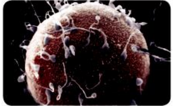
▲ شكل (١٩) الإخصاب
