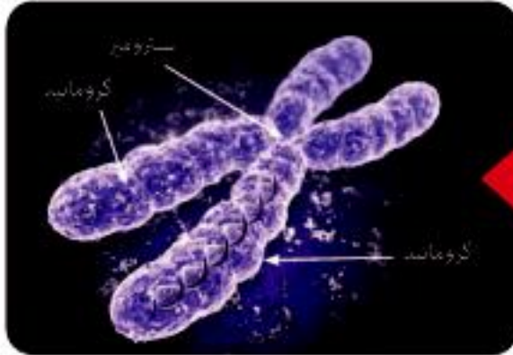
▲ شكل (٣) الكروموسوم
