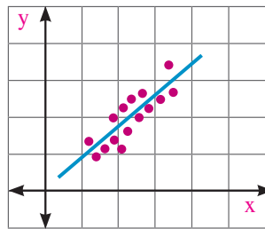
(2) Corrélation directe forte
