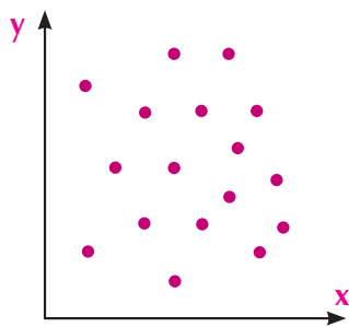
Figure 1 Pas de corrélation
