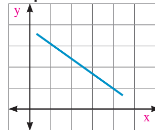
(6) Corrélation parfaite indirecte
