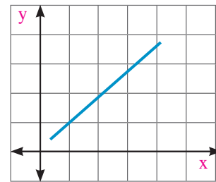
(3) Corrélation parfaite directe
