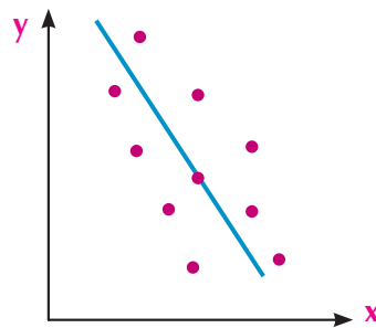
Figure 2 Corrélation linéaire indirecte (négative)
