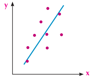
Figure 3 Corrélation linéaire directe (positive)
