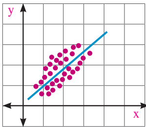
(1) Corrélation directe moyenne
