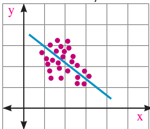
(4) Corrélation indirecte moyenne
