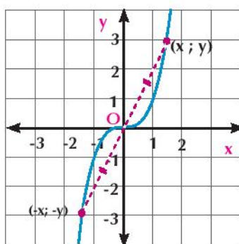
Symétrie par rapport à l'origine Fig (2)
