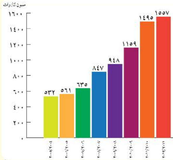
شكل (١٣): تطور إنتاج محطة كهرباء الزعفرانة.
