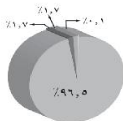
شكل (٦) توزيع موارد المياه في العالم.
