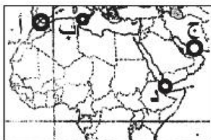
شكل ٢٨-١: التوزيع من المعادن بالوطن العربي
