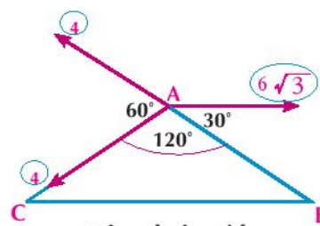
Triangle isocèle
