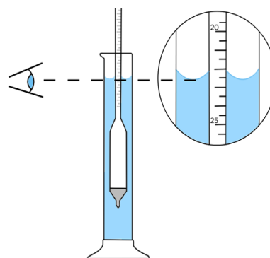
Figure (1-13) l'utilisation de l'Hydromètre
