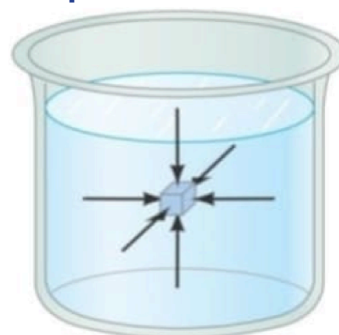
Figure (1-48) Les forces de pression sur un corps plongé dans un liquide
