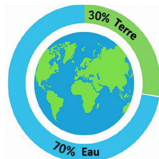
Figure ( 1-1 ) le pourcentage de l'atmosphère par rapport à l'hydrosphère sur la Terre
