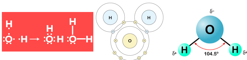
Figure (1-4) structure d'une molécule d'eau
