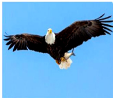
Figure (2) - (20) Courants de convection dans l'air
