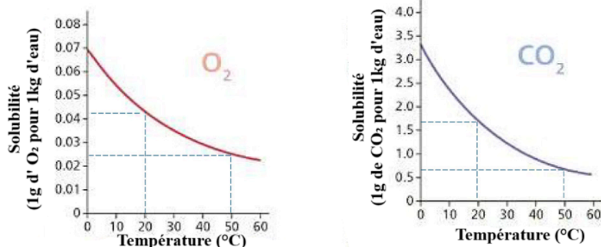
(Figure 1-40) Relation entre la solubilité des deux gaz \text{O}_2 et \text{CO}_2 dans l'eau et la température.
