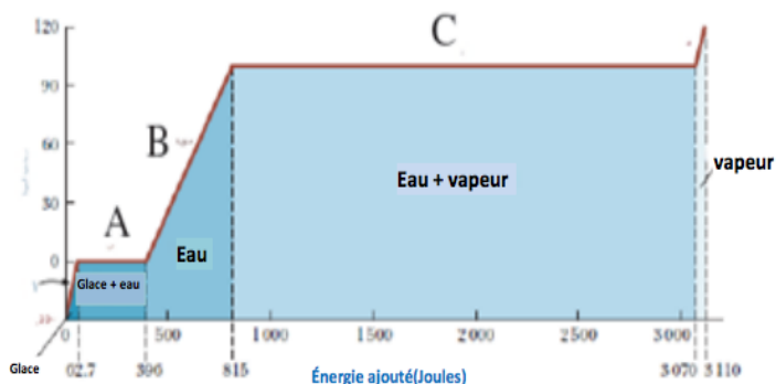
( Figure 1-20 ) la quantité de la chaleur que gagne l'eau lors de son chauffage
