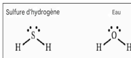
Figure 1-7) Molécule d'eau et molécule de sulfure d'hydrogène
