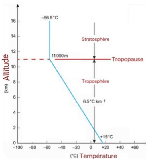
Figure (2-5) : La troposphère
