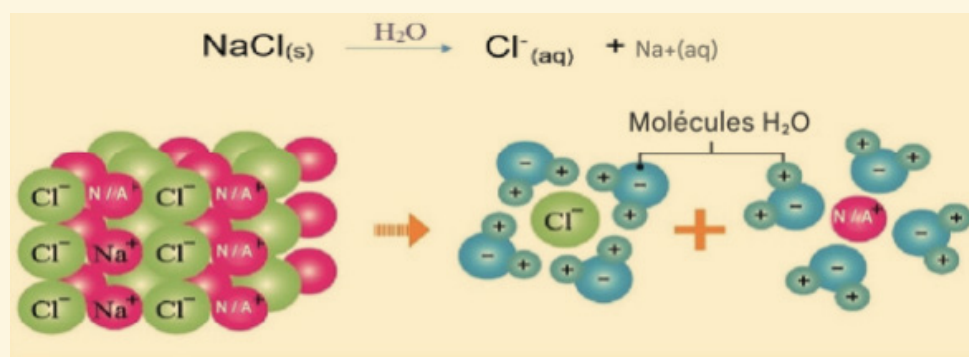
Figure (1-9) Dissociation du chlorure de sodium dans l'eau
