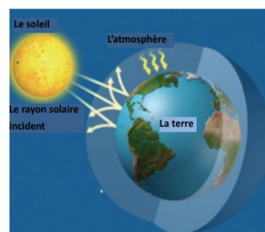
Figure (2-37) le réchauffement climatique
