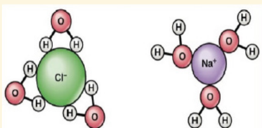
(Figure 1-8) Ions chlorure et sodium dans l'eau
