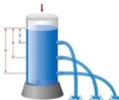
Figure (1-49) Variation de la pression en fonction de la profondeur
