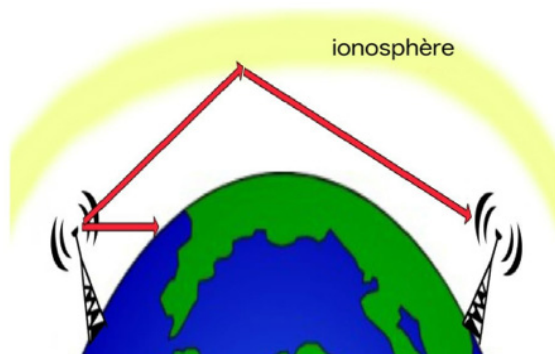
Figure (2-7) : l'ionosphère
