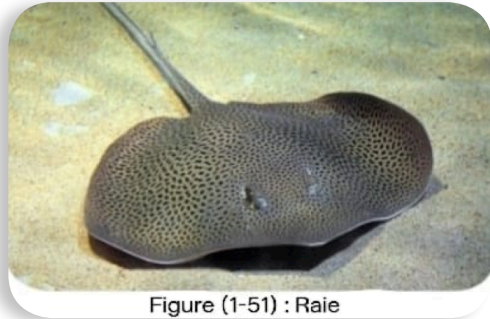
Figure (1-51) : Raie
