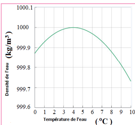
Figure (1-11) le changement de la densité de l'eau avec la température
