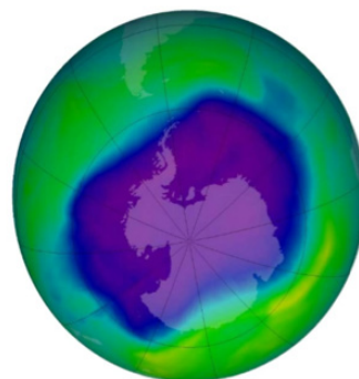
Figure (2-15) : Trou dans la couche d'ozone
