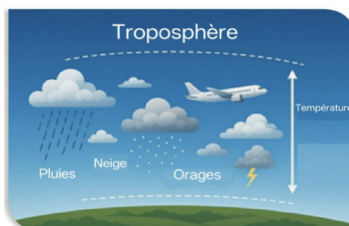
Figure (2-4) La troposphère
