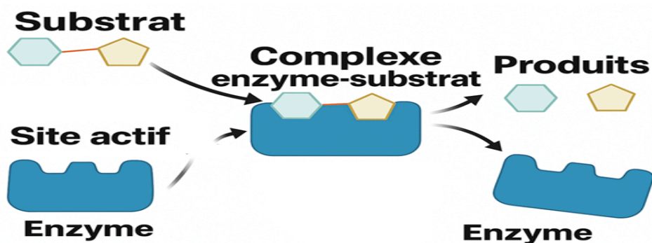
(Figure 1-28) : Enzyme en tant que catalyseur
