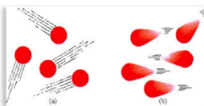
Figure (2-11) : Mouvement des molécules de gaz
