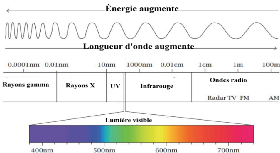
(Figure 1-44) : Le spectre électromagnétique
