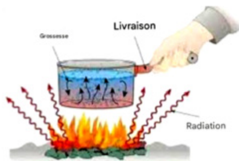
Figure (2) - (19) Mécanismes de transfert de chaleur
