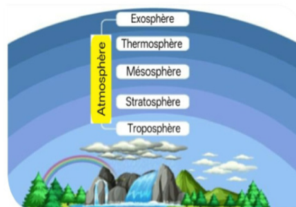
Figure (2-3) Les couches de l'atmosphère
