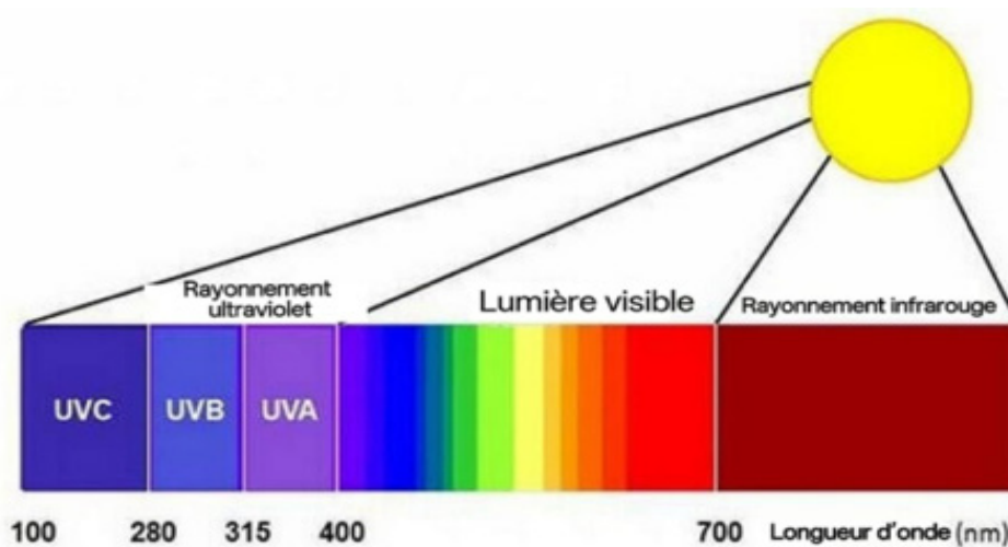
Figure (2 - 13) : Les types de rayonnements ultraviolets
