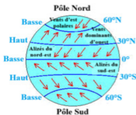
Figure (2-30) – Les systèmes de vents
