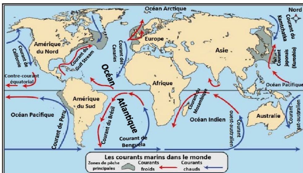
Figure (1-14) les courants d'eau dans les océans
