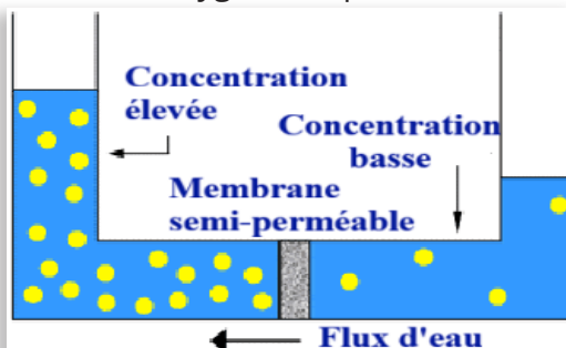
Figure (1-36) la pression osmotique
