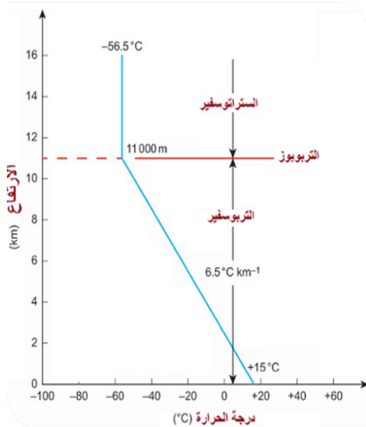
الشكل (5-2) التروبوسفير
