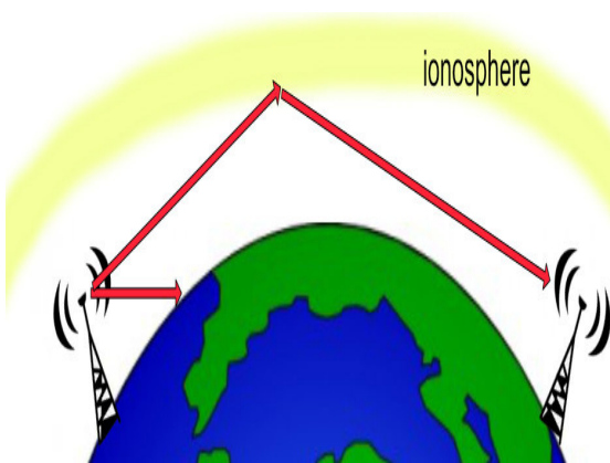
الشكل (2-7) الأيونوسفير
