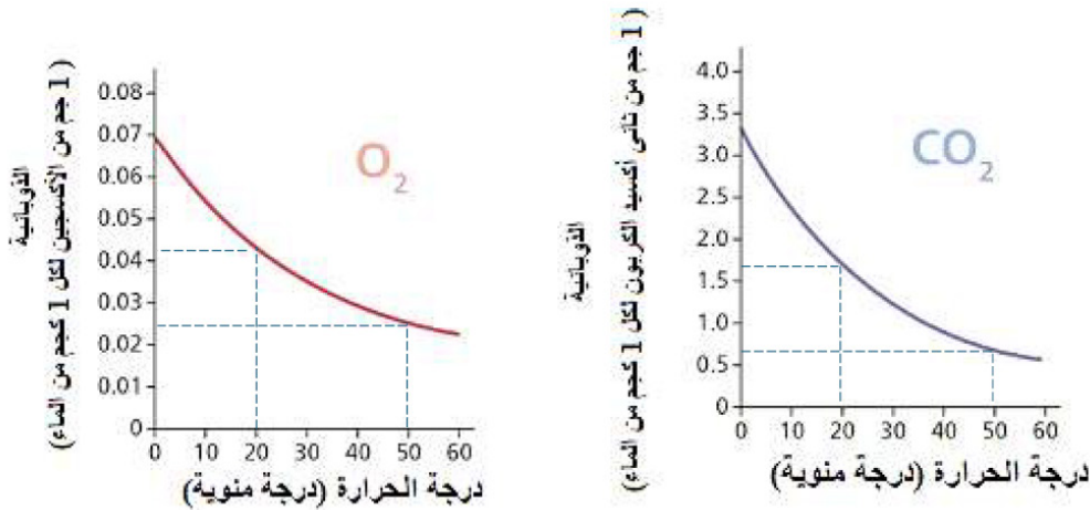
(الشكل 1 - 40) العلاقة بين ذوبانية \text{O}_2 ، \text{CO}_2 في الماء ودرجة الحرارة
