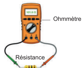
Figure (25) Mesure de la résistance
