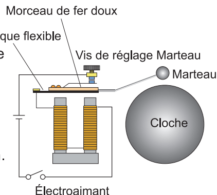
Figure (4) Schéma du circuit de la sonnette électrique
