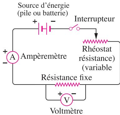
Figure (1) Circuit de la loi d'Ohm
