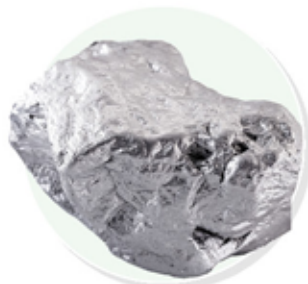
معدن الكروم
