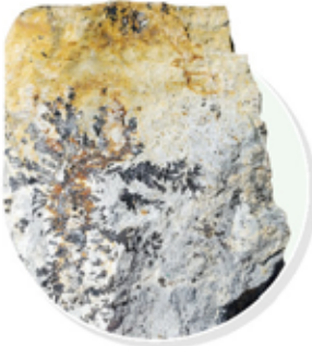
خام المنجنيز
