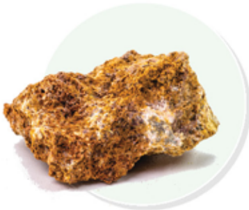
خام البوكسيت
