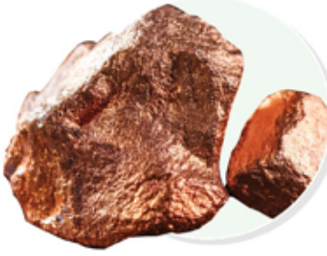
خام النحاس
