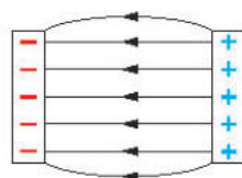
Figure (15) Lignes de forces électriques entre deux plaques métalliques chargées avec des charges différentes
