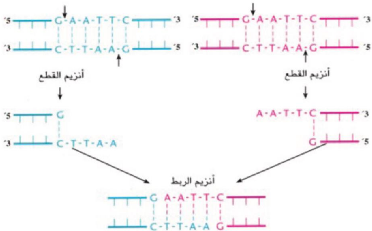
(شكل ٤) دور انزيمات القص والربط في قطع وربط قطعتين مختلفتين من DNA عند مواقع محددة
