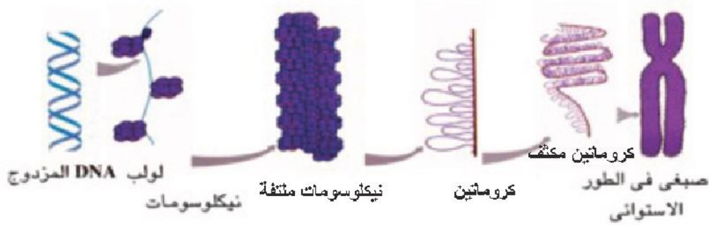
شكل (ب) خطوات تكثيف الـ DNA فى حقيقيات النواة
