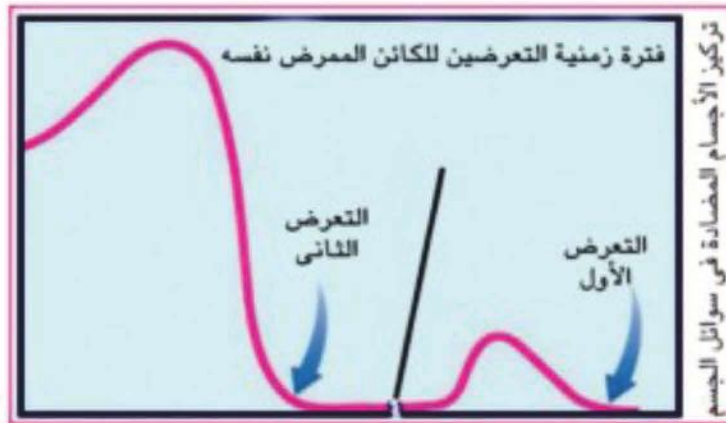
شكل (٢١) الاستجابة المناعية الأولية والثانوية
