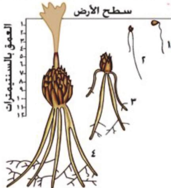
شكل (١٢) حركة الشد فى الجذور لأبصال النرجس
